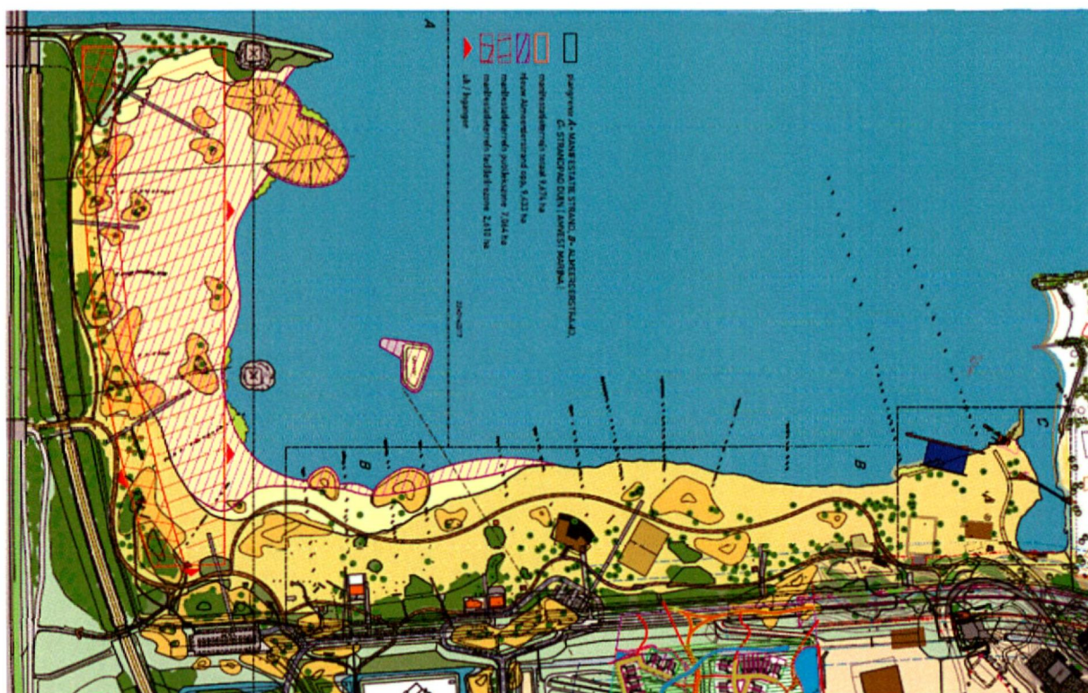
Figuur 5 Almeerderstrand toekomstige inrichting
